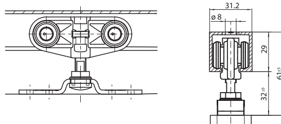
Vozík so závesnou skrútkou
