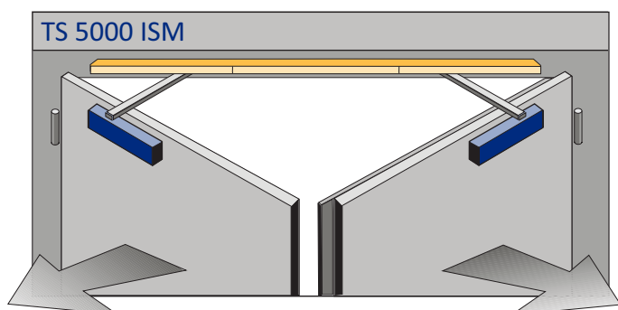
Montáž systému ISM na strane závesov
