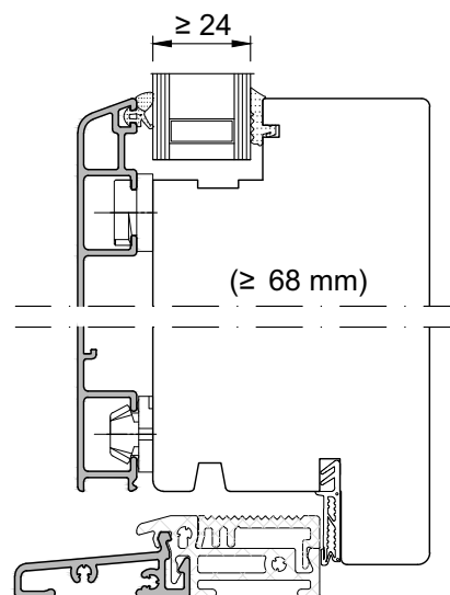
P 47-50 K Plastový adaptér na prerušenie tepelného mosta
