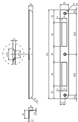
Protiplech oblý s nosom B00590.37
