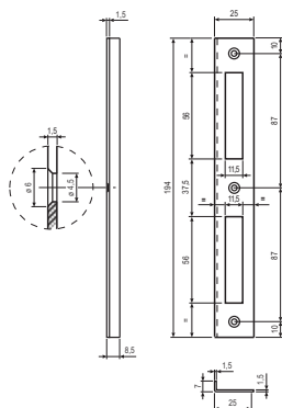
Protiplech rovný - oblý B00590.42
