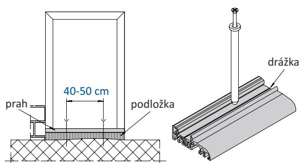
Montáž univerzálnou podložkou
