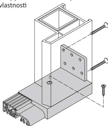
Montáž univerzálnou podložkou
